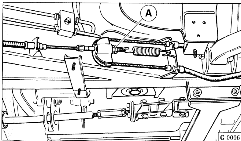
Fig. 9 - Regolazione freno a mano.
