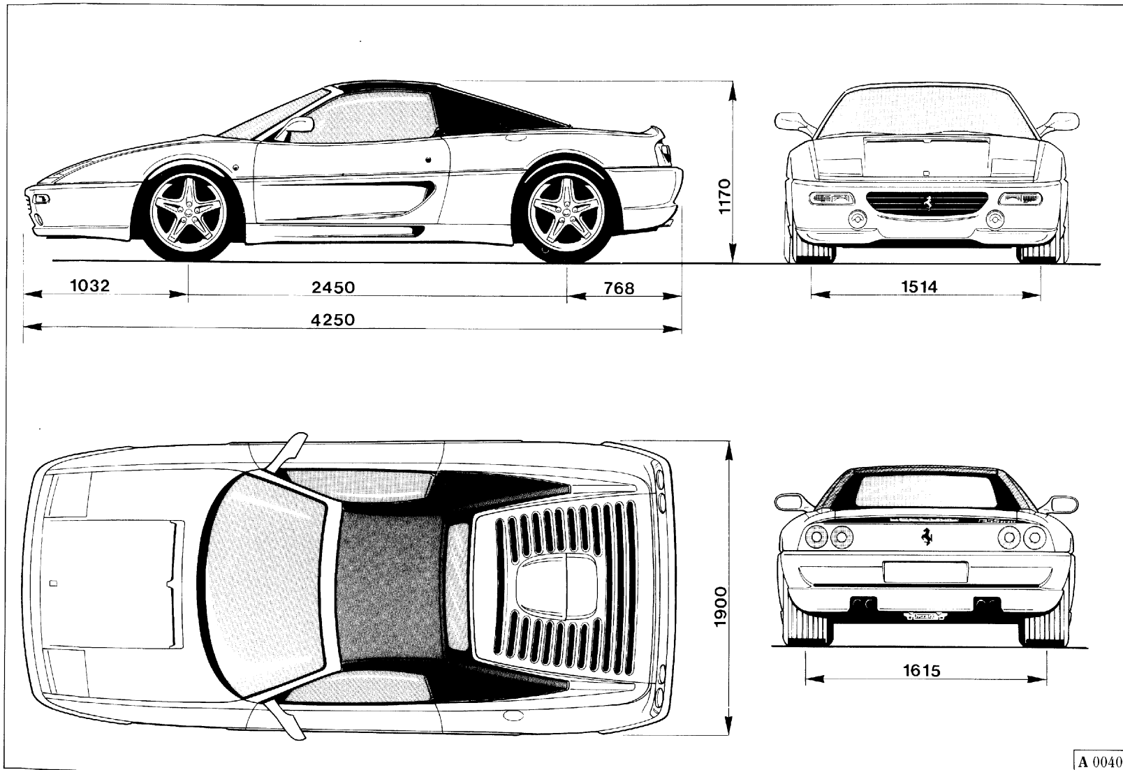
Fig. 2 - Dimensioni vettura.
