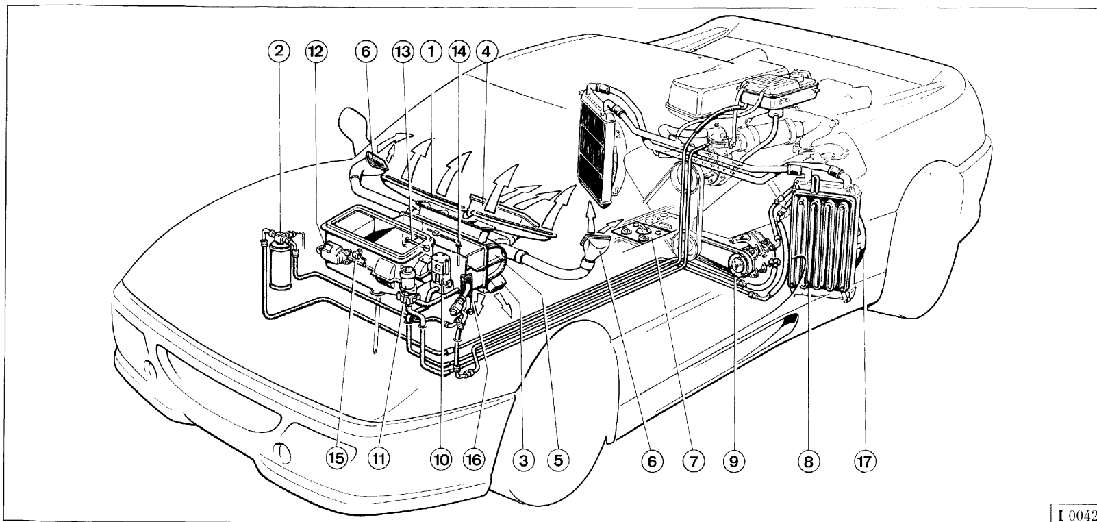
Fig. 1 - Impianto climatizzazione
