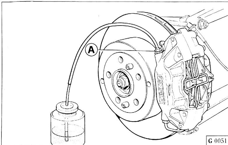
Fig. 6 - Disaerazione dei cilindretti freni
