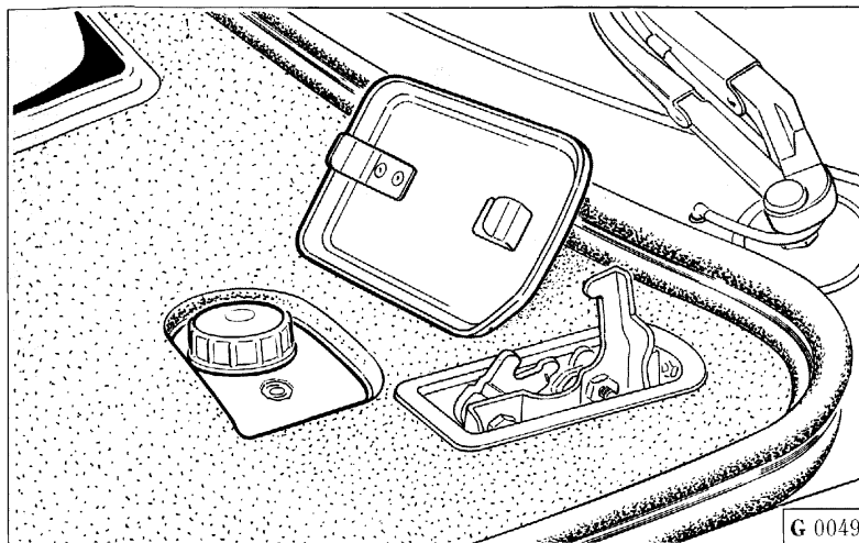
Fig. 4 - Serbatoio liquido comando freni
