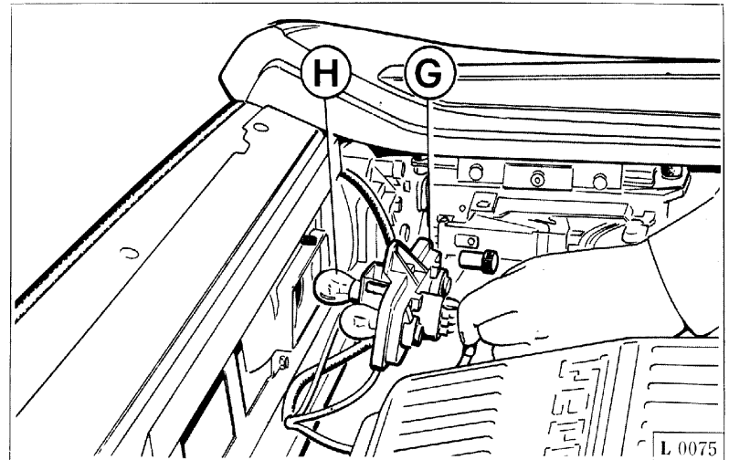
Fig. 13 - Remplacement de l'ampoule feu arrière
