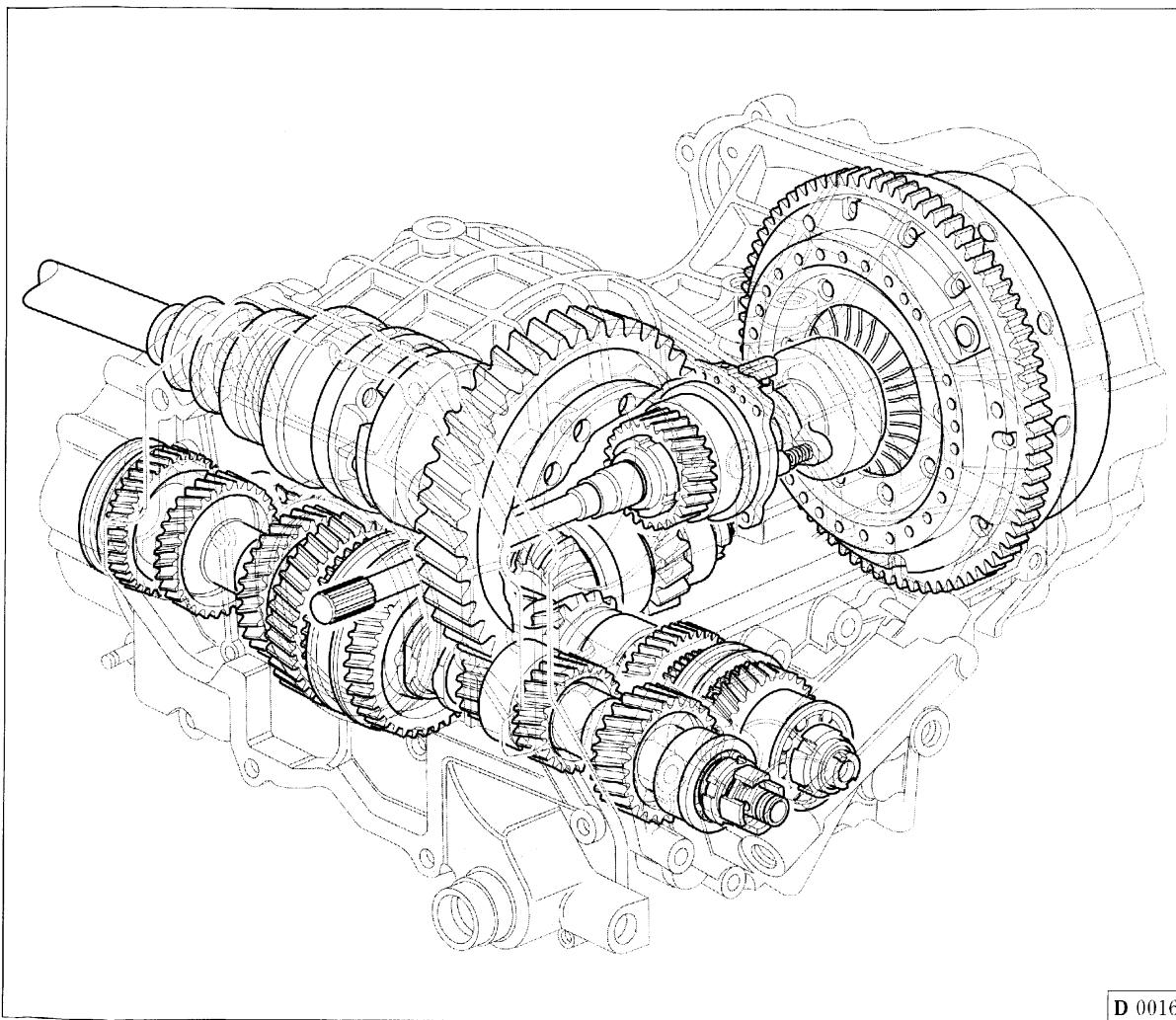
Fig. 4 - Complesivo frizione, cambio e differenziale.
