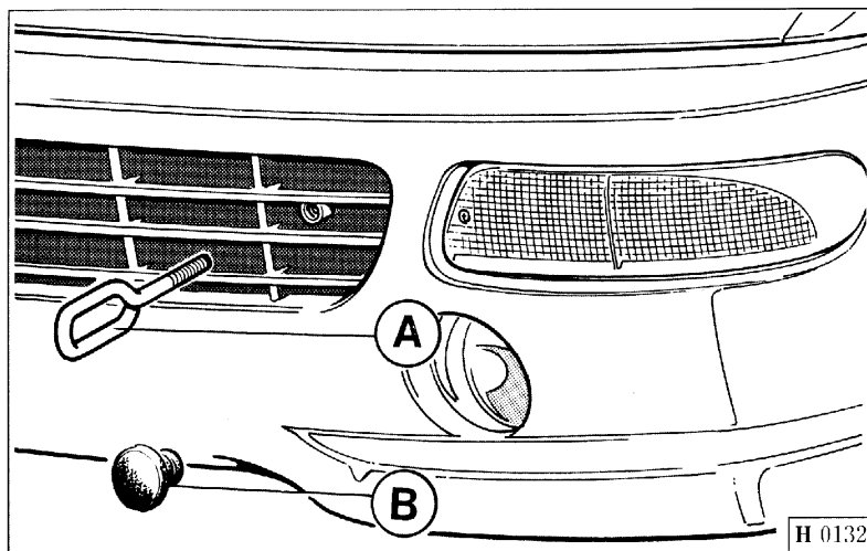
Fig. 37 - Posizione sede gancio di traino.
