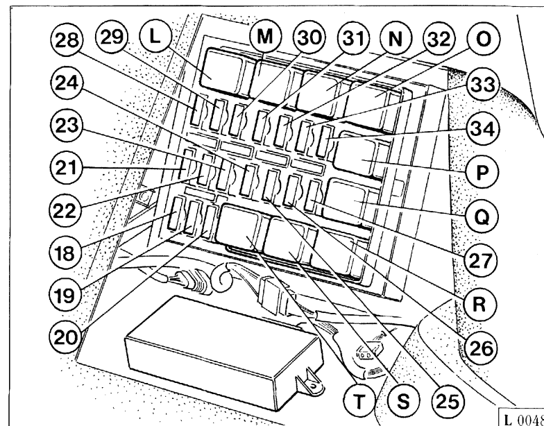
Fig. 15 - Centralina elettrica sotto appoggiapiedi passeggero.
