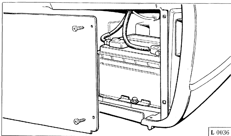
Fig. 1 - Posizione batteria.
