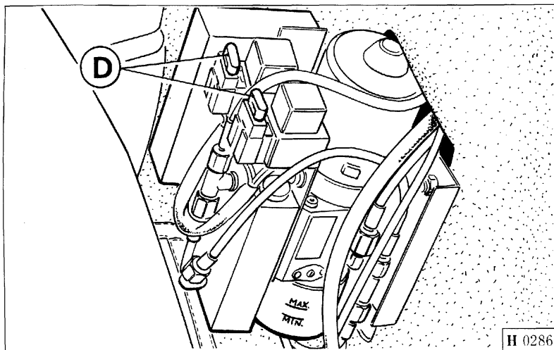
Fig. 36 - Posizione fusibili.
