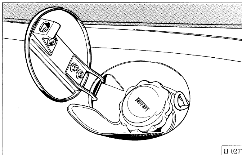
Fig. 29 - Fuel filler cap
