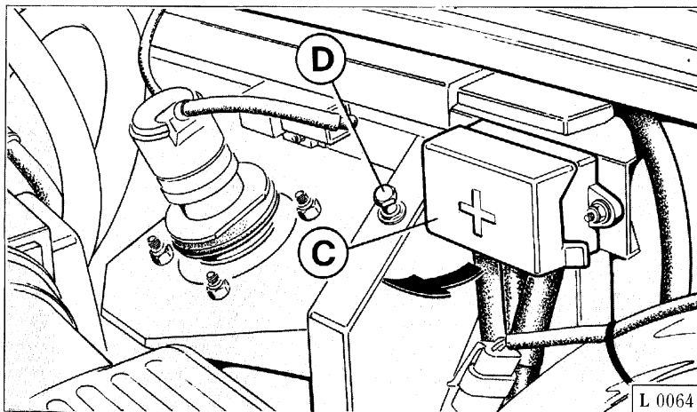
Fig. 4 - Blocchetto per ricarica batteria C - Positivo batteria; D - Massa.
