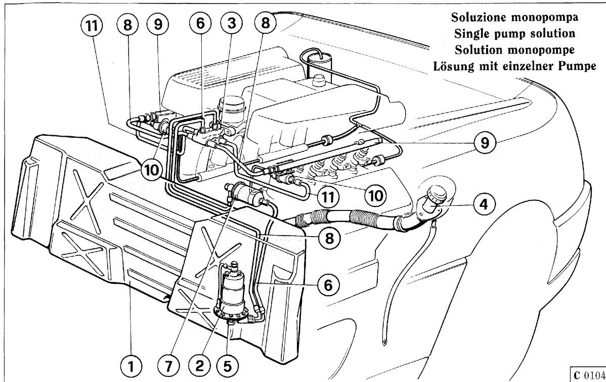
Fig. 3 - Impianto alimentazione benzina
