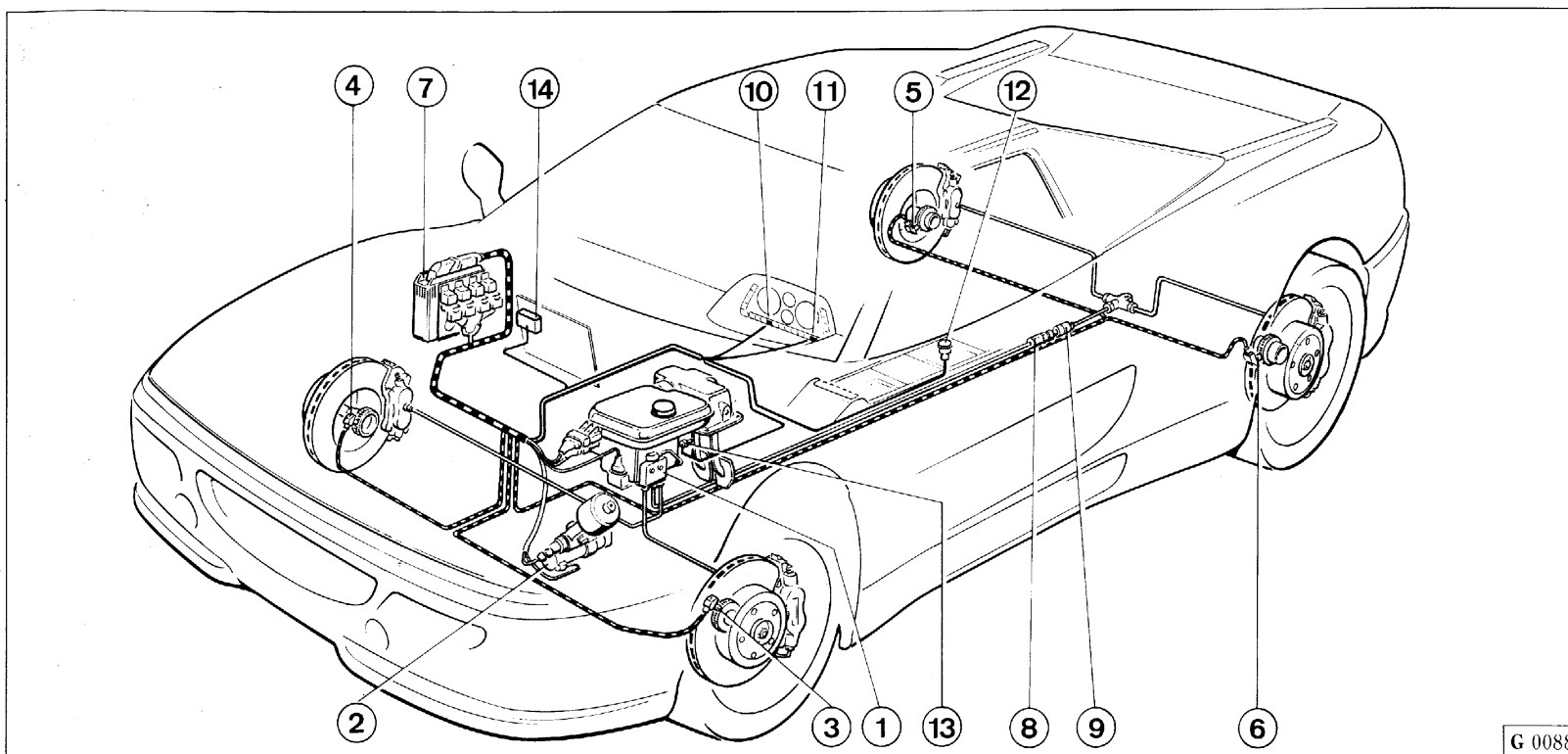
Fig. 1 - Impianto freni
