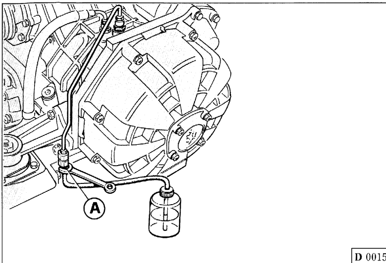
Fig. 3 - Spurgo aria
