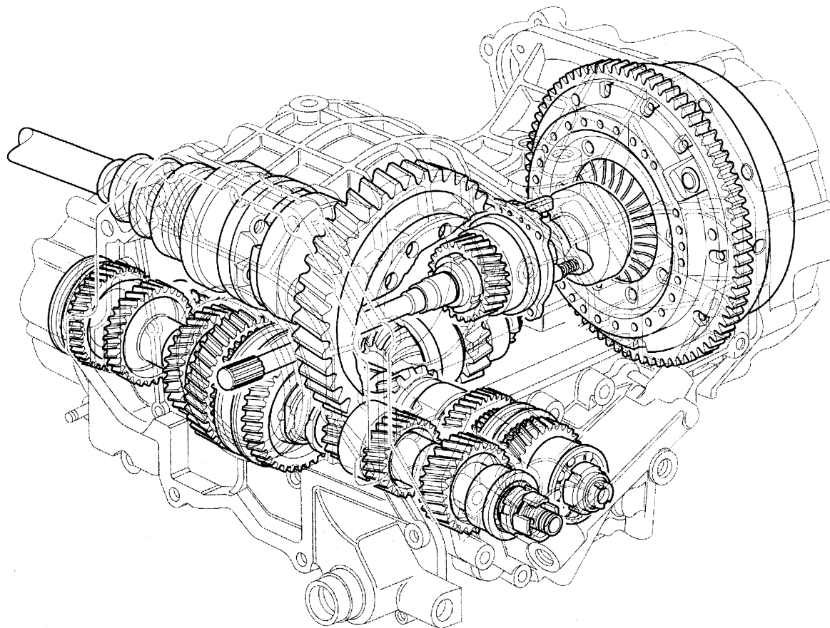
Fig. 4 - Complesso frizione, cambio e differenziale.
