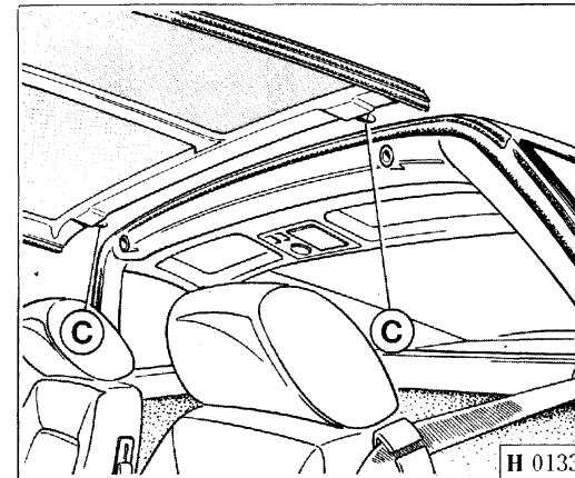
Fig. 37 - Démontage/remontage du toit rigide.
