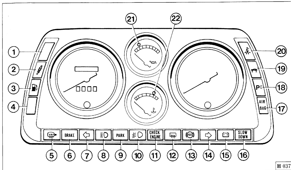
Fig. 2 - Segnalatori luminosi.
