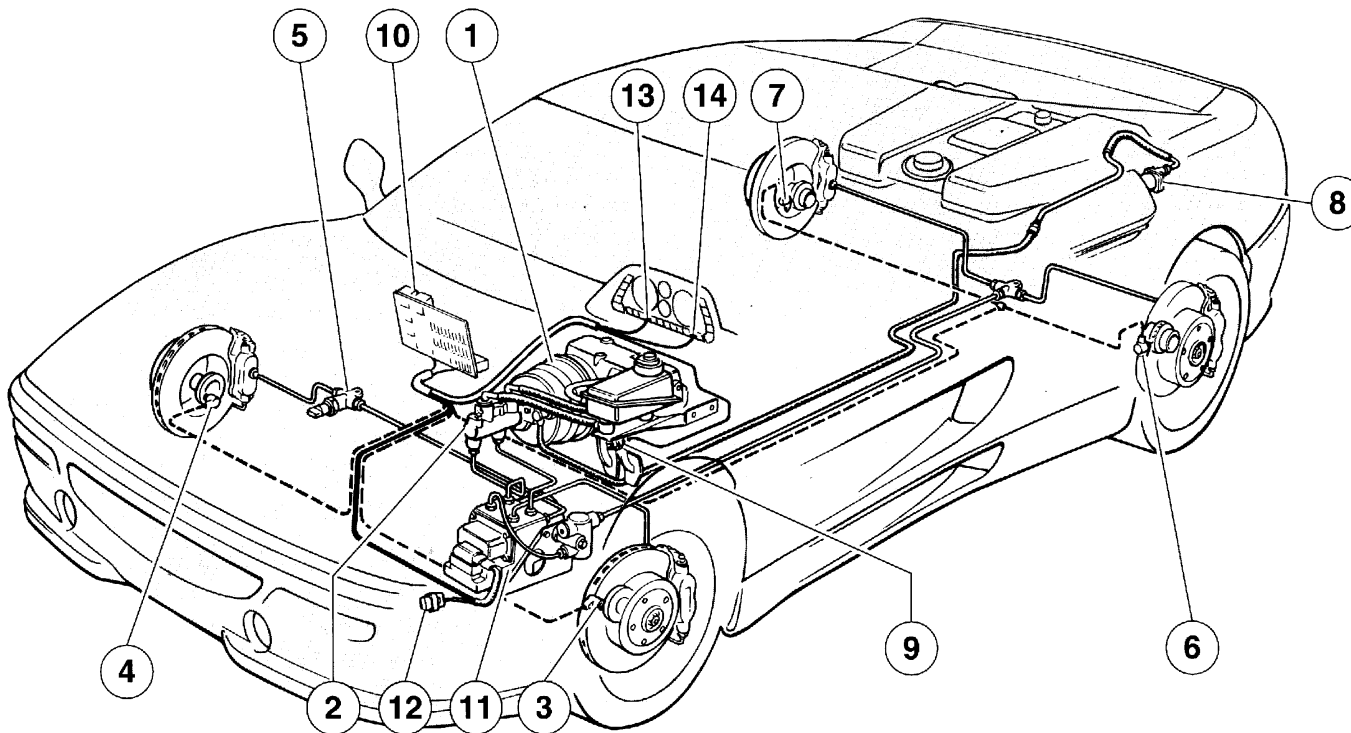
Fig. 3 - Impianto freni
