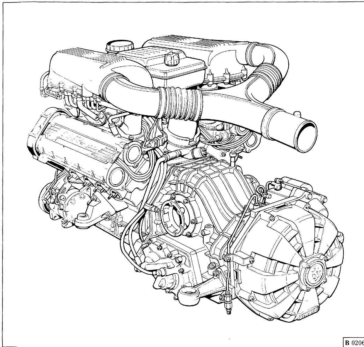
Fig. 1 - Gruppo motopropulsore.
