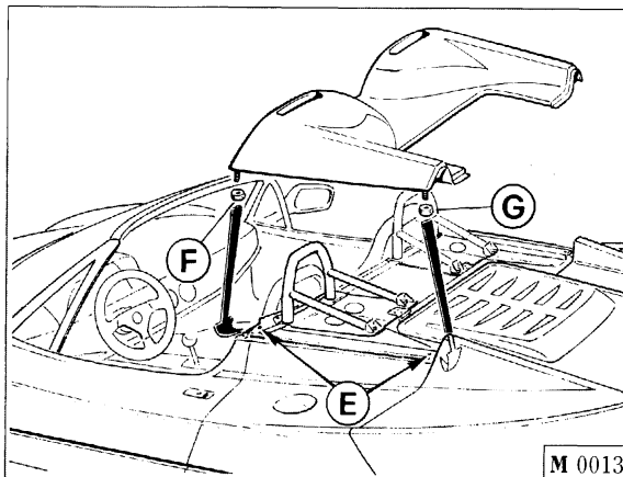
Fig. 20 - Fissaggio roll-bar.
