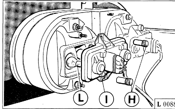
Fig. 11 - Sostituzione lampada F - Dadi di fissaggio - G - Protezione; H - Vite; I - Portalamпада; L - Lampada.
