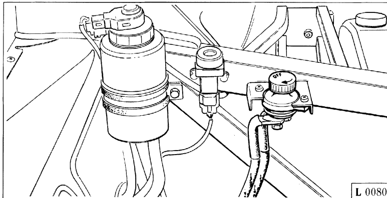
Fig. 2 - Interruttore staccabatteria.
