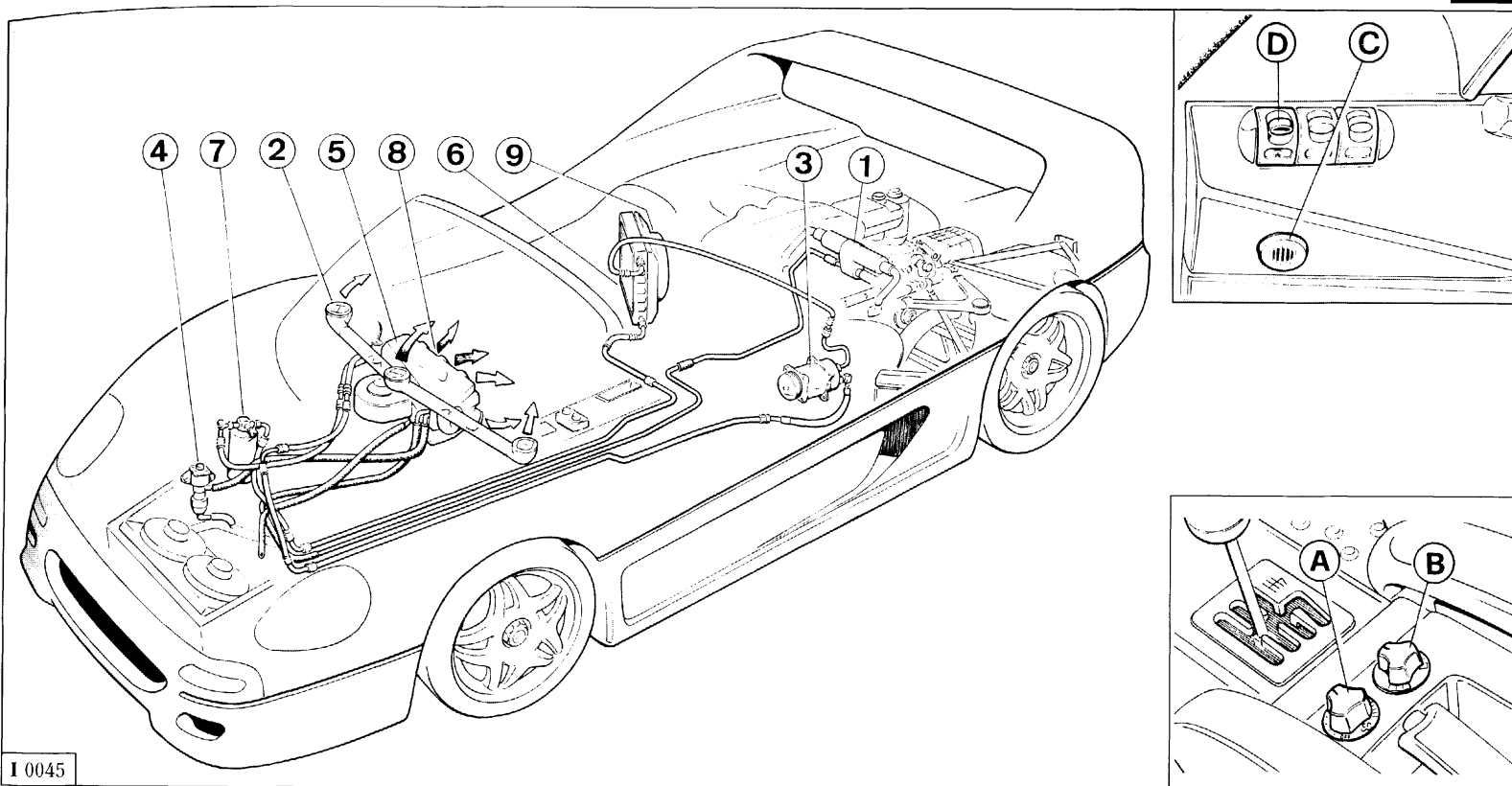
Fig. 27 - Impianto climatizzazione
