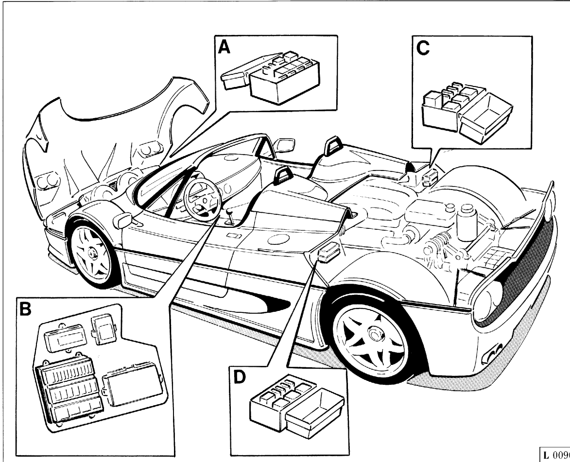
Fig. 13 - Posizione centraline elettriche A - Centralina anteriore; B - Centralina sotto appoggiapiedi lato passeggero; C - Centralina posteriore Dx.; D - Centralina posteriore Sx.
