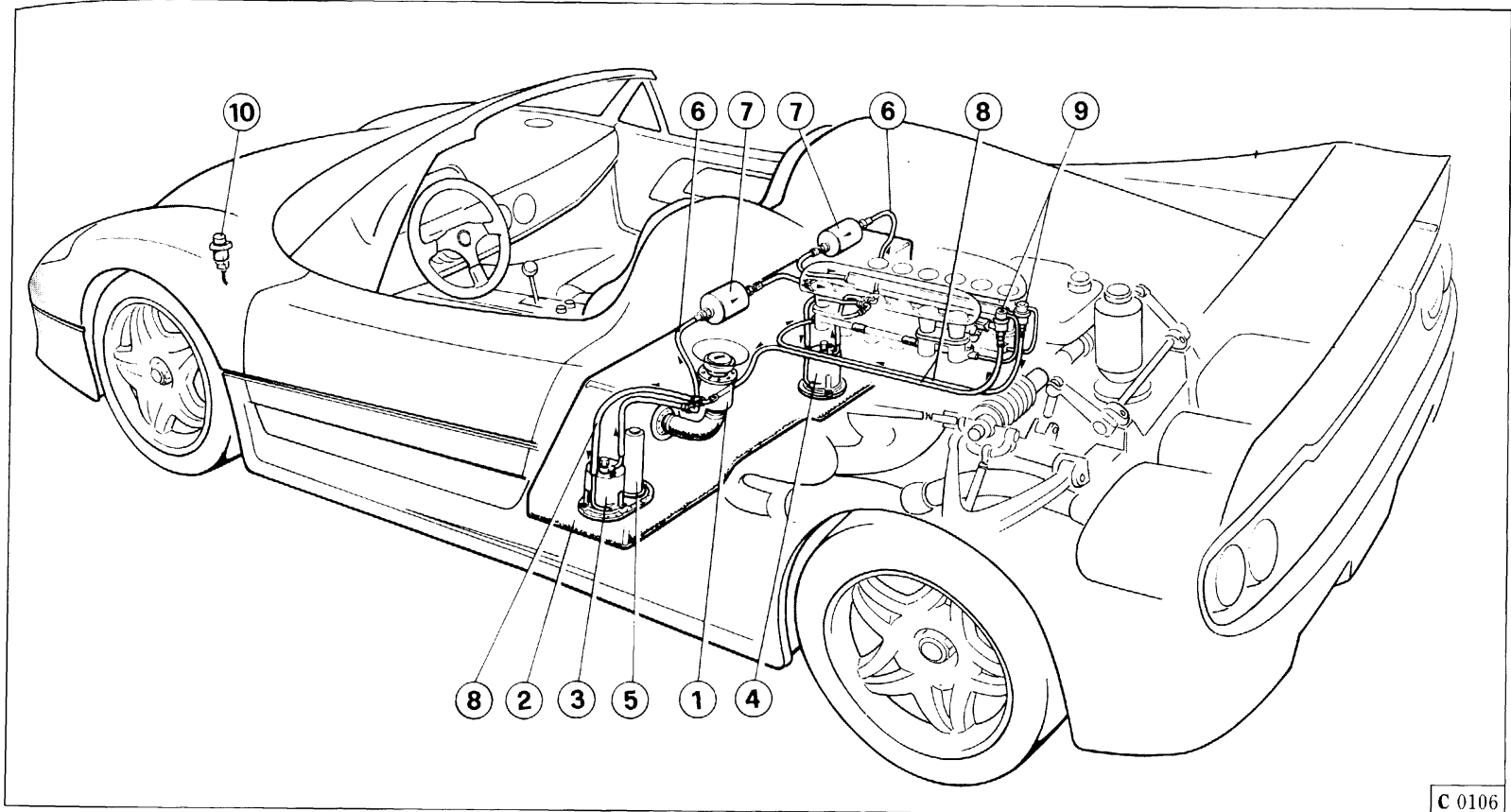
Fig. 11 - Impianto alimentazione benzina 1 - Bocchettone di carico; 2 - Serbatoio carburante; 3 - Pompa benzina Sx; 4 - Pompa benzina Dx; 5 - Indicatore livello carburante; 6 - Tubazione di mandata benzina; 7 - Filtro benzina; 8 - Tubazione di riflusso benzina; 9 - Regolatore pressione carburante; 10 - Interruttore inerziale.
