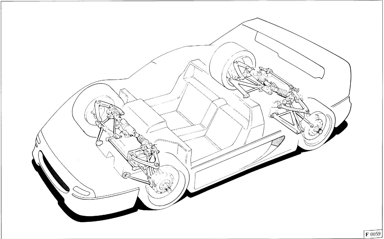
Abb. 13 - Darstellung der Vorder- und Hinteraufhängung.
