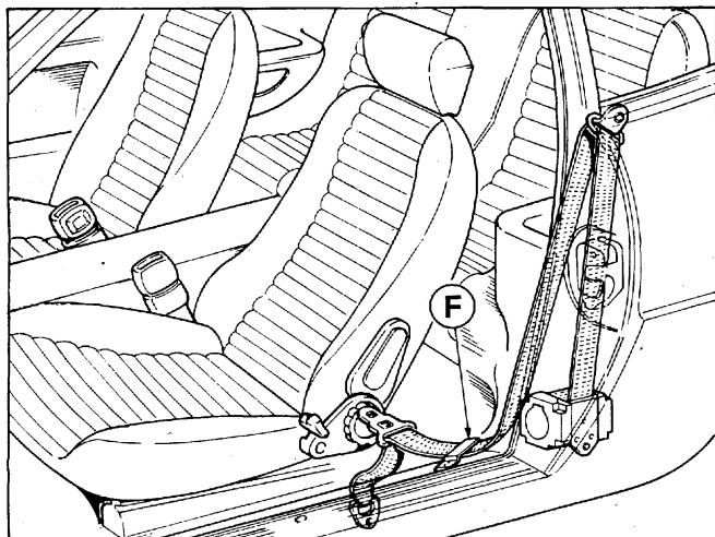
19) Gancio di fermo per cintura a riposo.
