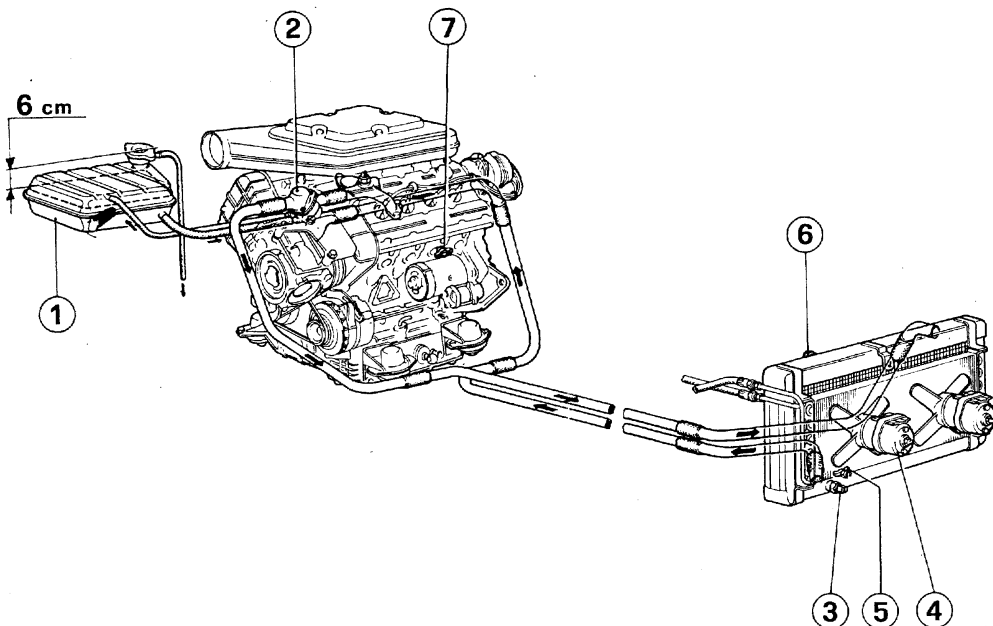
46) Cooling system layout.
