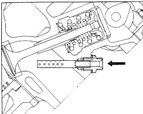
65) Air injection nozzle.
