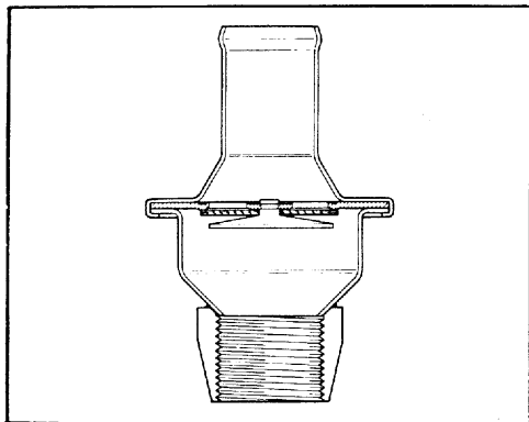
66) Check valve.
