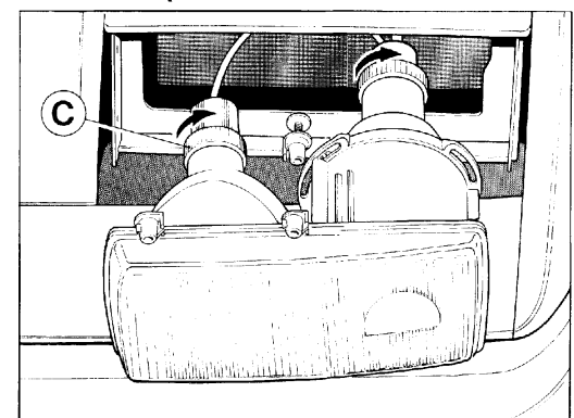
4) Remplacement de l'ampoule du projecteur
