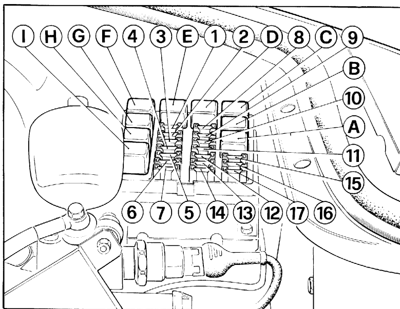
Fig. 10 - Centrale électrique coffre à bagages
