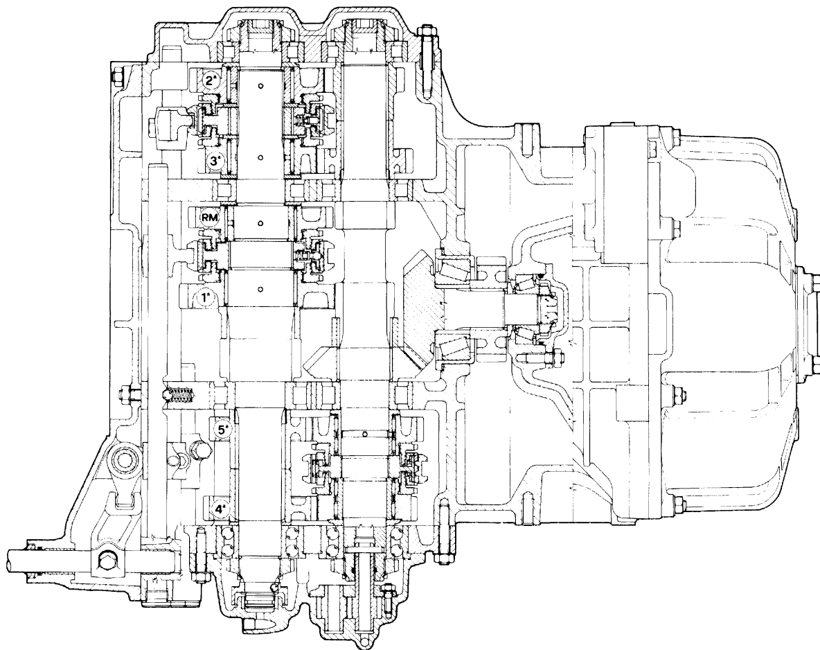
Fig. 4 - Complesso frizione - cambio - differenziale
