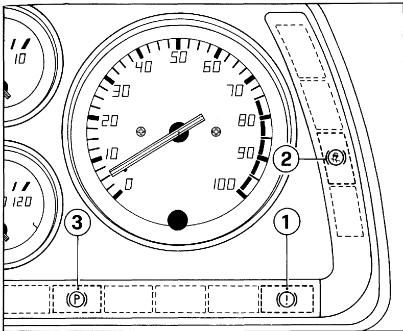
Fig. 2 - Spie freni
