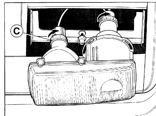
4) Scheinwerferbirnen - Austausch
