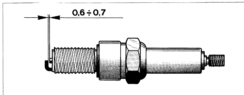
Fig. 4 - Controllo distanza elettrodi
