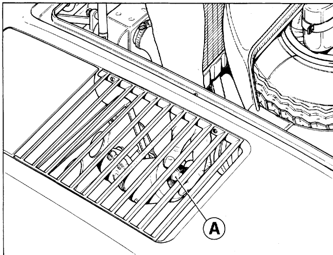
84) Headlamp lifting motor.
