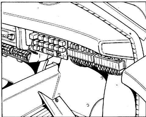
33) Fuses box position. 33) Posizione quadro elettrico.
