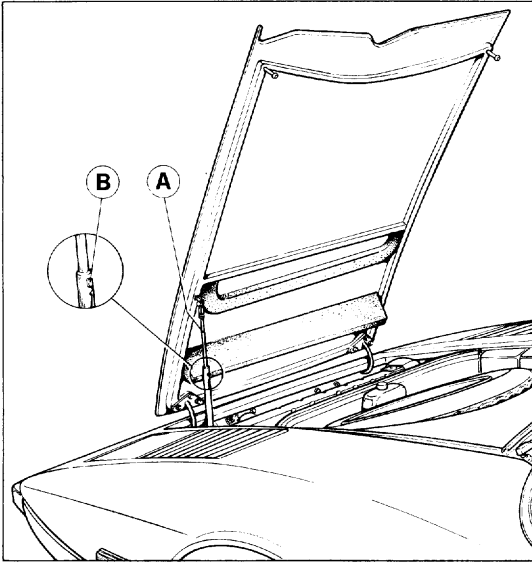
39) Front bonnet.
