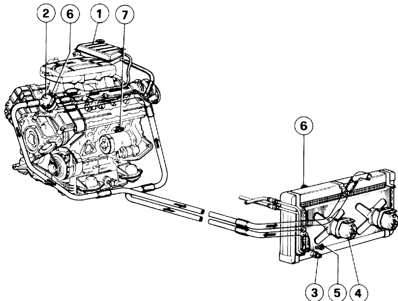
54) Cooling system layout.
