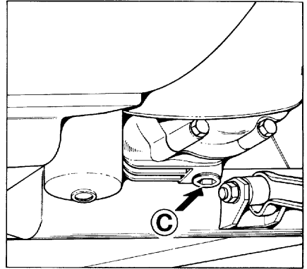
72) Oil drain plug from the clutch housing. 72) Tappo scarico olio dalla campana frizione.
