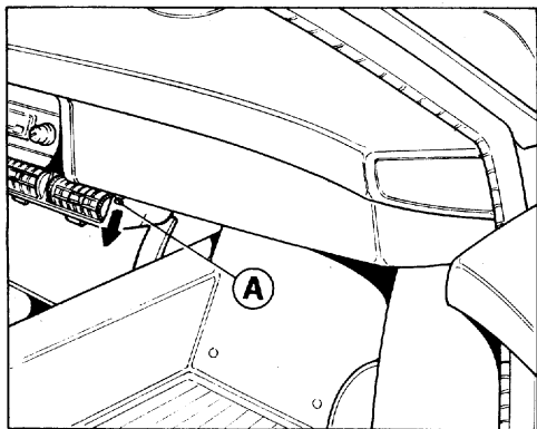
32) Removing the cover. 32) Smontaggio coperchio.
