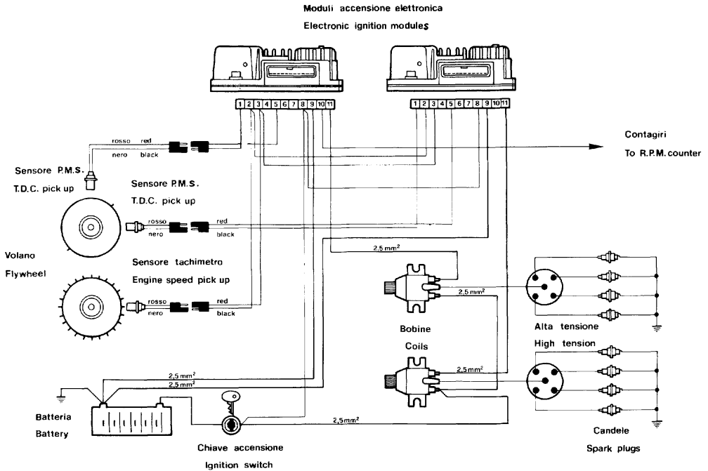
62) Schema del circuito di accensione.
