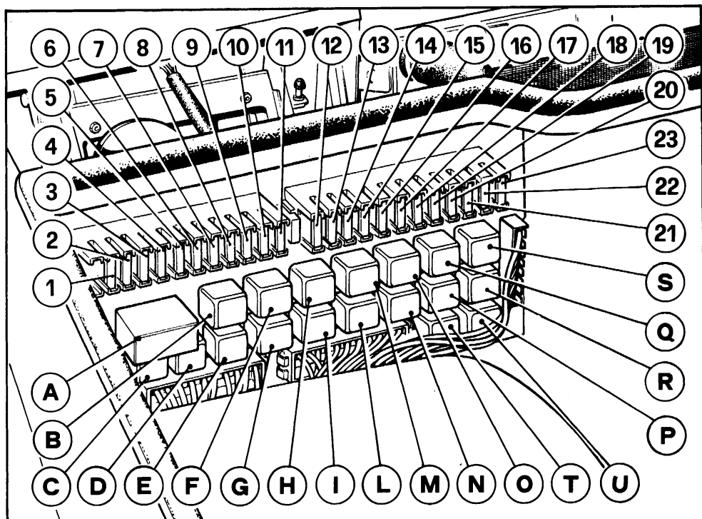
85) Valvole fusibili e teleruttori
