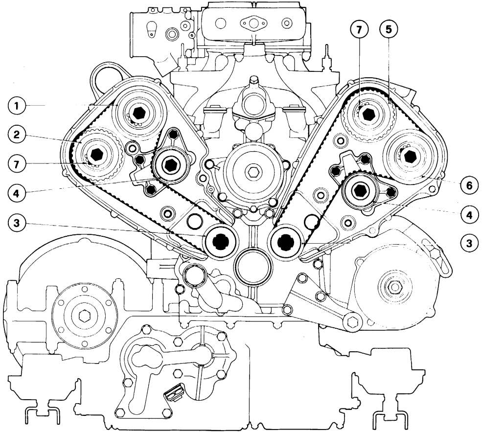
47) Schema comando distribuzione
