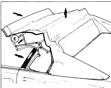
Figg. 94-95 - Apertura capote E - Traversina mobile
