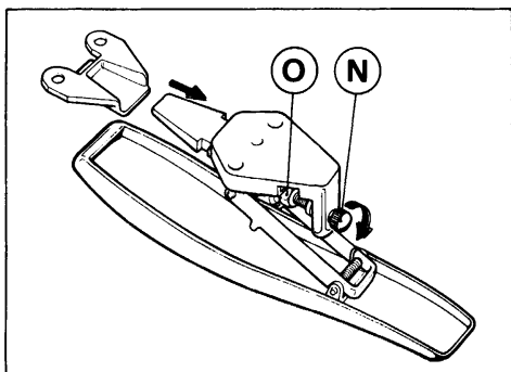
100) Regastro filettato (N) con dado di bloccaggio (O) per regolare la tensione della capote
