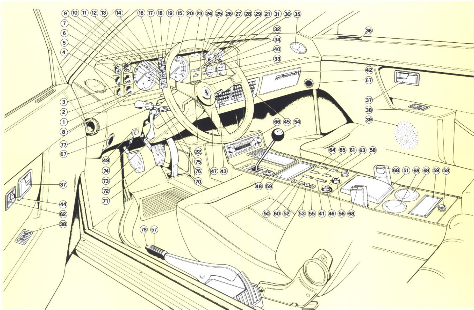
10) Apparecchi di controllo e comandi. 10) Commandes et appareils de contrôle. 10) Instruments and controls.
