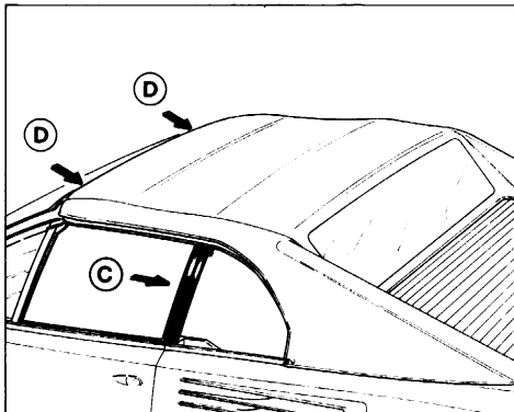
93) Apertura capote C - Montante laterale; D - Centraggio capote.
