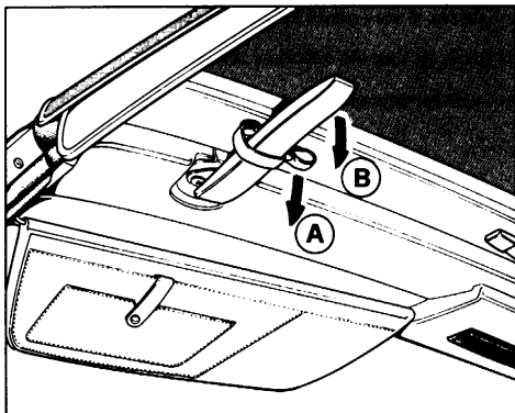
92) Sbloccaggio capote A - Cinghie di sicurezza; B - Maniglia di sbloccaggio.
