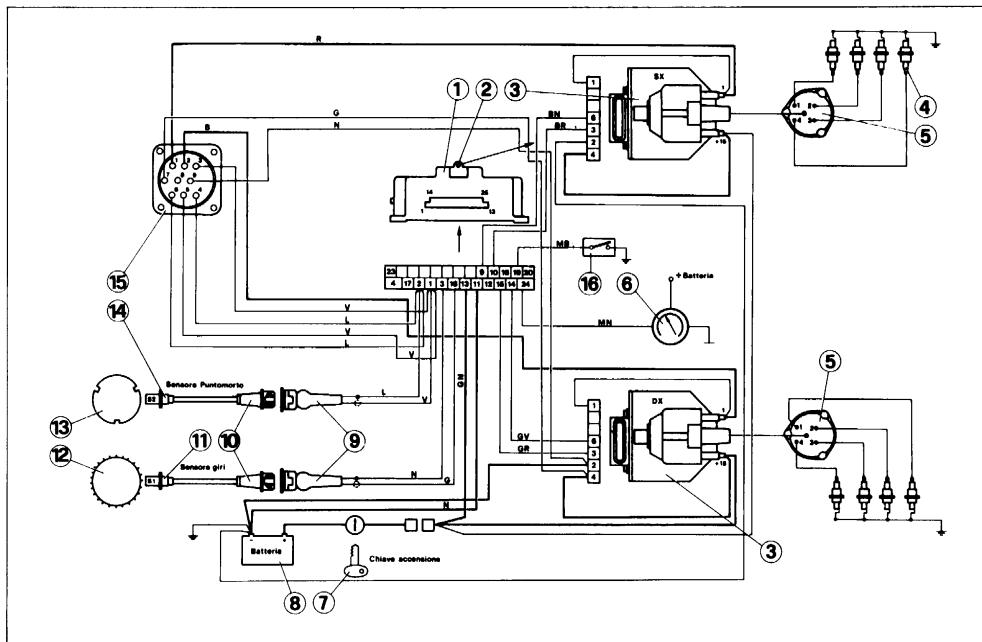
Fig. 56 - Circuito accensione
