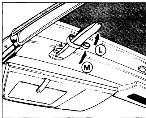
99) Chiusura capote L - Maniglia bloccaggio capote; M - Cinghia di sicurezza
