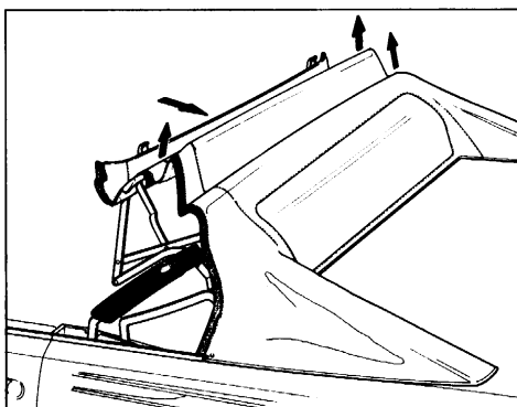
Figg. 94-95 Ouverture de la capote E - Traverse mobile
