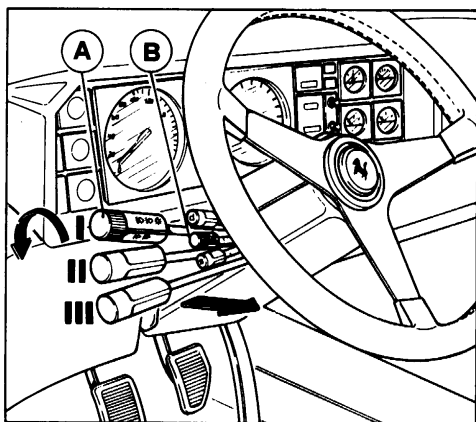
15) High/low beam and direction indicator control levers 15) Leve di commutazione
