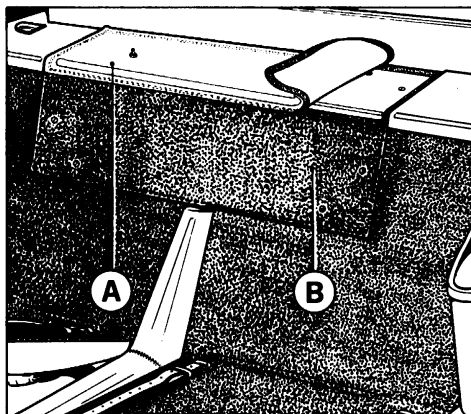
107) Accesso al motore dall'interno vettura A - Protezione; B - Paratia.
